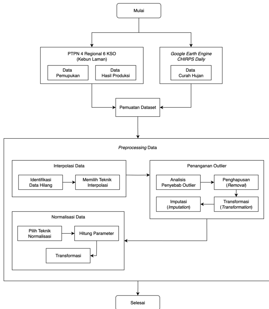
Gambar 3. 23 Desain Pengelolaan Data
