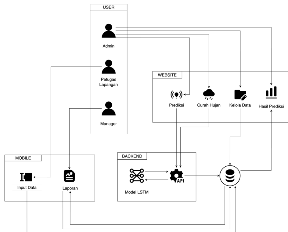
Gambar 3. 10 Arsitektur Umum Sistem Prediksi Hasil Produksi
