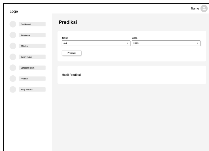
Gambar 3. 19 Interface Prediksi
